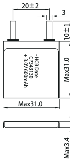
Dimensions in mm (GB1804-m)
