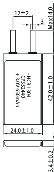
Dimensions in mm (GB1804-m)
