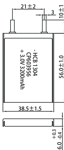
Dimensions in mm (GB1804-m)
