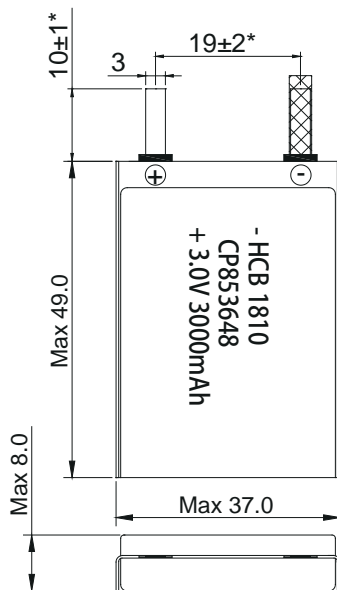
Dimensions in mm (GB1804-m)
