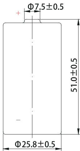
Dimensions in mm (GB1804-m)
