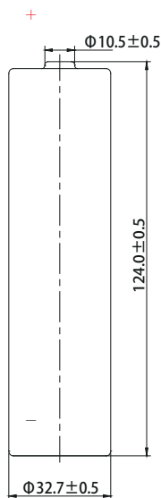
Dimensions in mm (GB1804-m)
